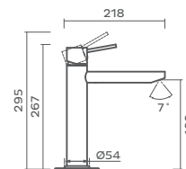
Cano alto (25cm) High spout (25cm) ◊ Pied surélevé (25cm)
