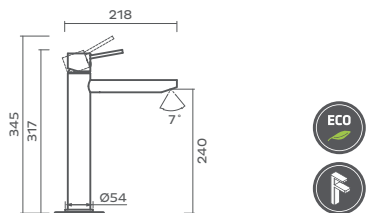
Cano alto (30cm) High spout (30cm) ◊ Pied surélevé (30cm)
