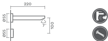
2 Águas Mixed water inlet ◊ Eau mélangée
