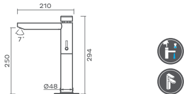
2 Águas Mixed water inlet ◊ Eau mélangée
