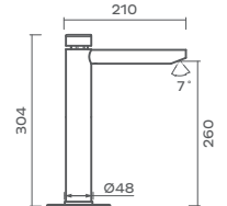
1 Água One water inlet ◊ Une entrée d'eau
