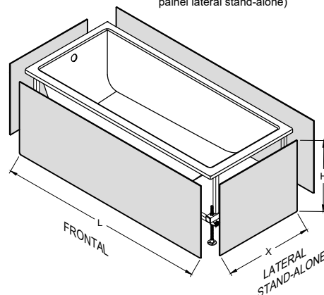
APLICAÇÃO STAND-ALONE (Painel frontal + painel lateral stand-alone)
