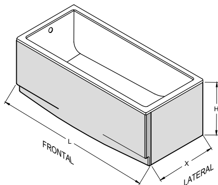
APLICAÇÃO DE CANTO (Painel frontal+painel lateral)
