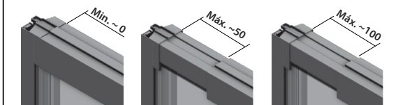
L2E - MARGEM DE AFINACÃO 1000 = 0-50 MM / 1100-1800 = 0-100 MM
