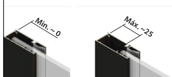
LF - MARGEM DE AFINAÇÃO = 0-25 MM
