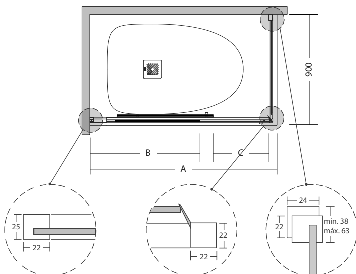
L2E - MARGEM DE AFINACÃO 1000 = 0-50 MM / 1100-1800 = 0-100 MM
